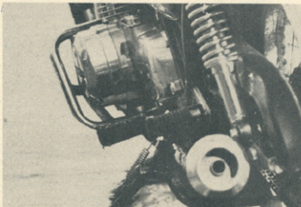
Pri hitri športni vožnji drsajo po asfaltu stojalo motorja, stopalke in naknadno montiran ščitnik alternatorja
